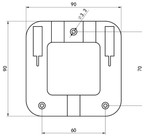
安装底座尺寸（单位：mm）
